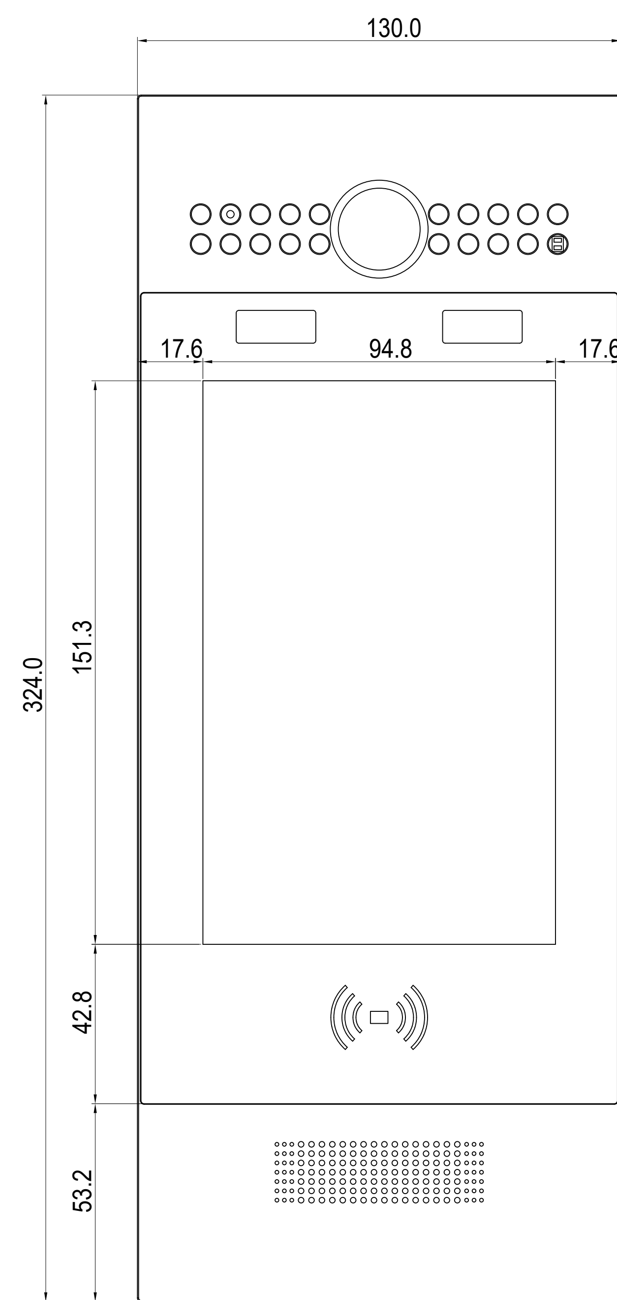
① 正视图
