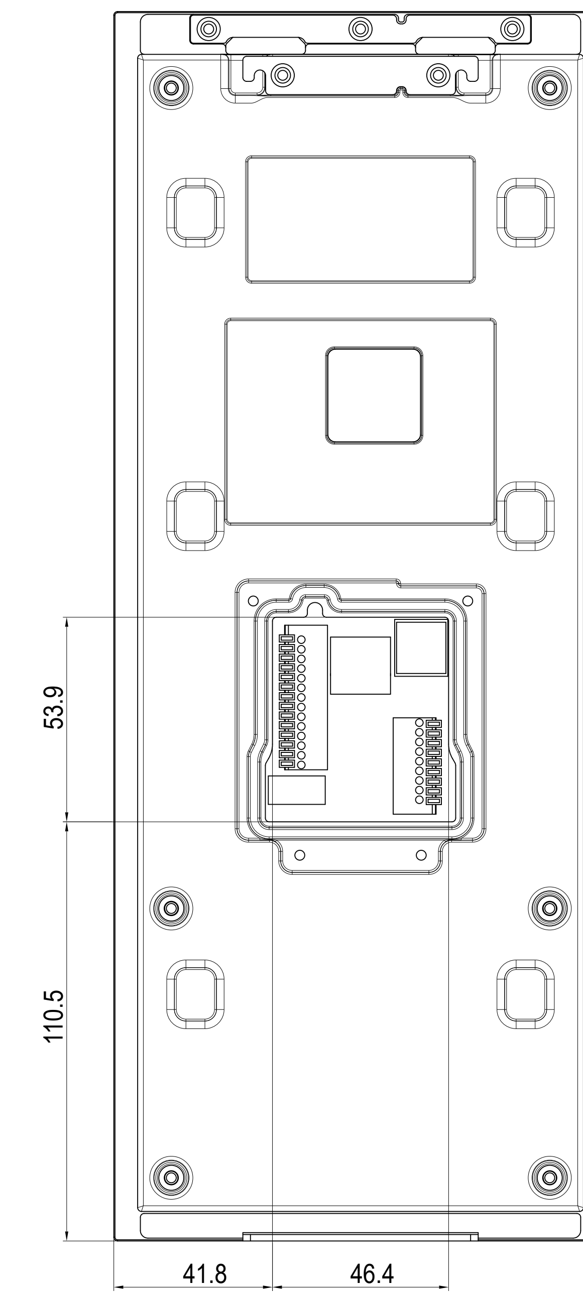
④ 后视图
