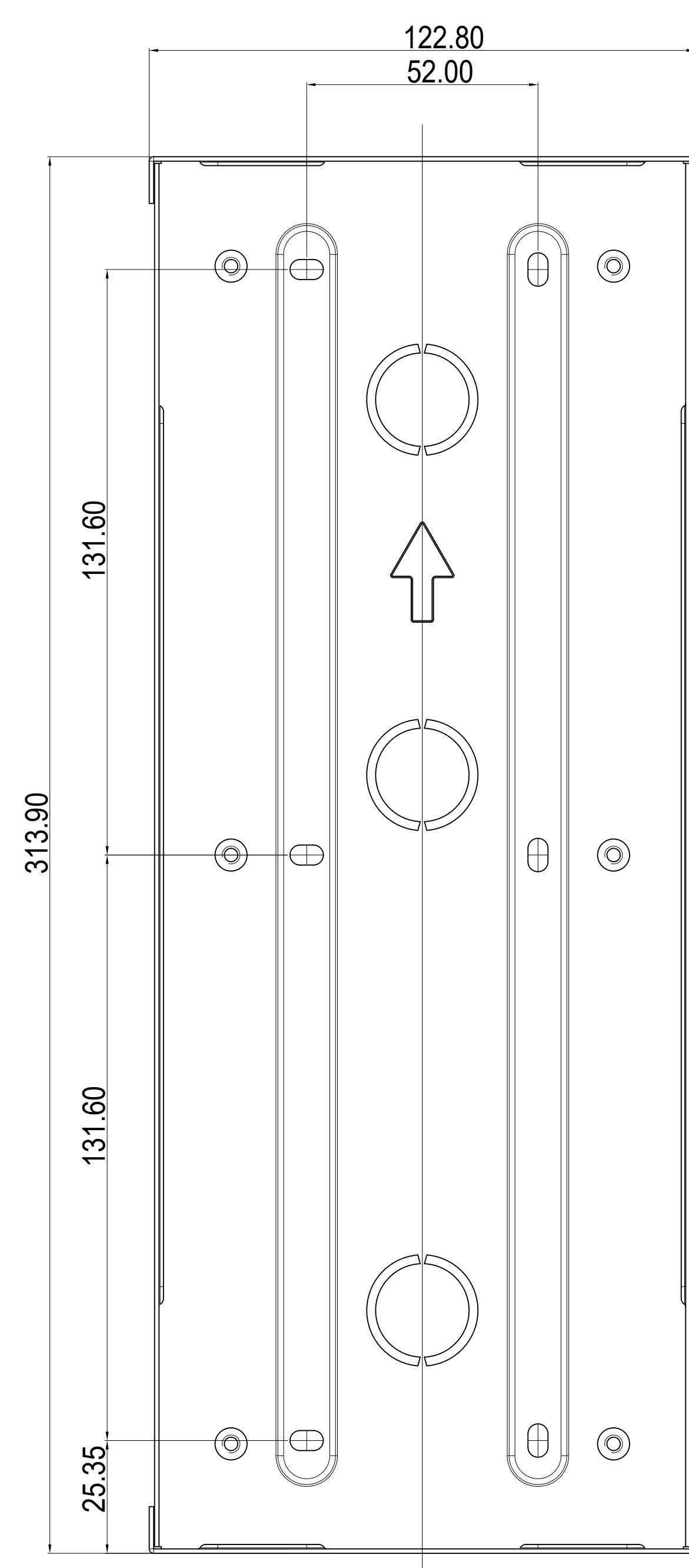
① 正视图
